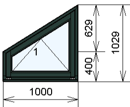
Pos. 8, 1 St.
