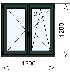
Pos. 13, 1 St.
