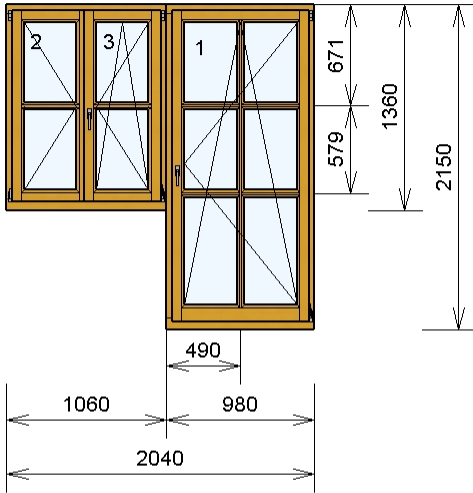
Pos. 5, 1 St.
