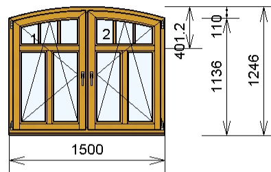
Pos. 15, 1 St.
