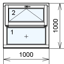
Pos. 15, 1 St.
