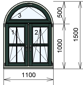
Pos. 3, 1 St.
