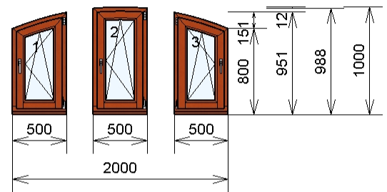
Pos. 12, 1 St.
