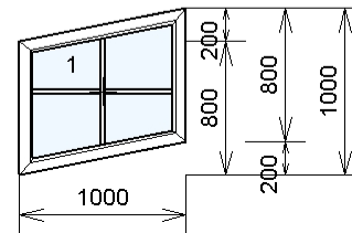
Pos. 7, 1 St.
