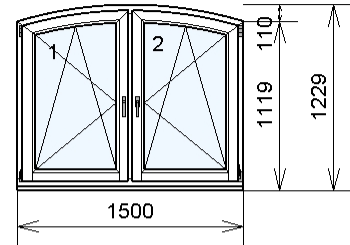
Pos. 4, 1 St.
